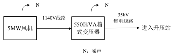
图 4-1 建设项目运营期产污节点
