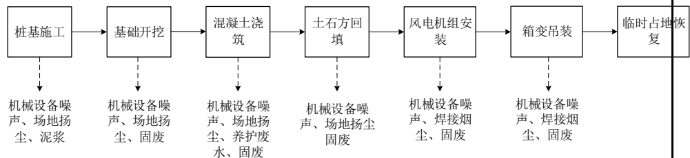
图 2-5 风电、箱变施工产污节点图
