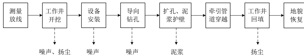
图 2-7 拉管施工示意图
