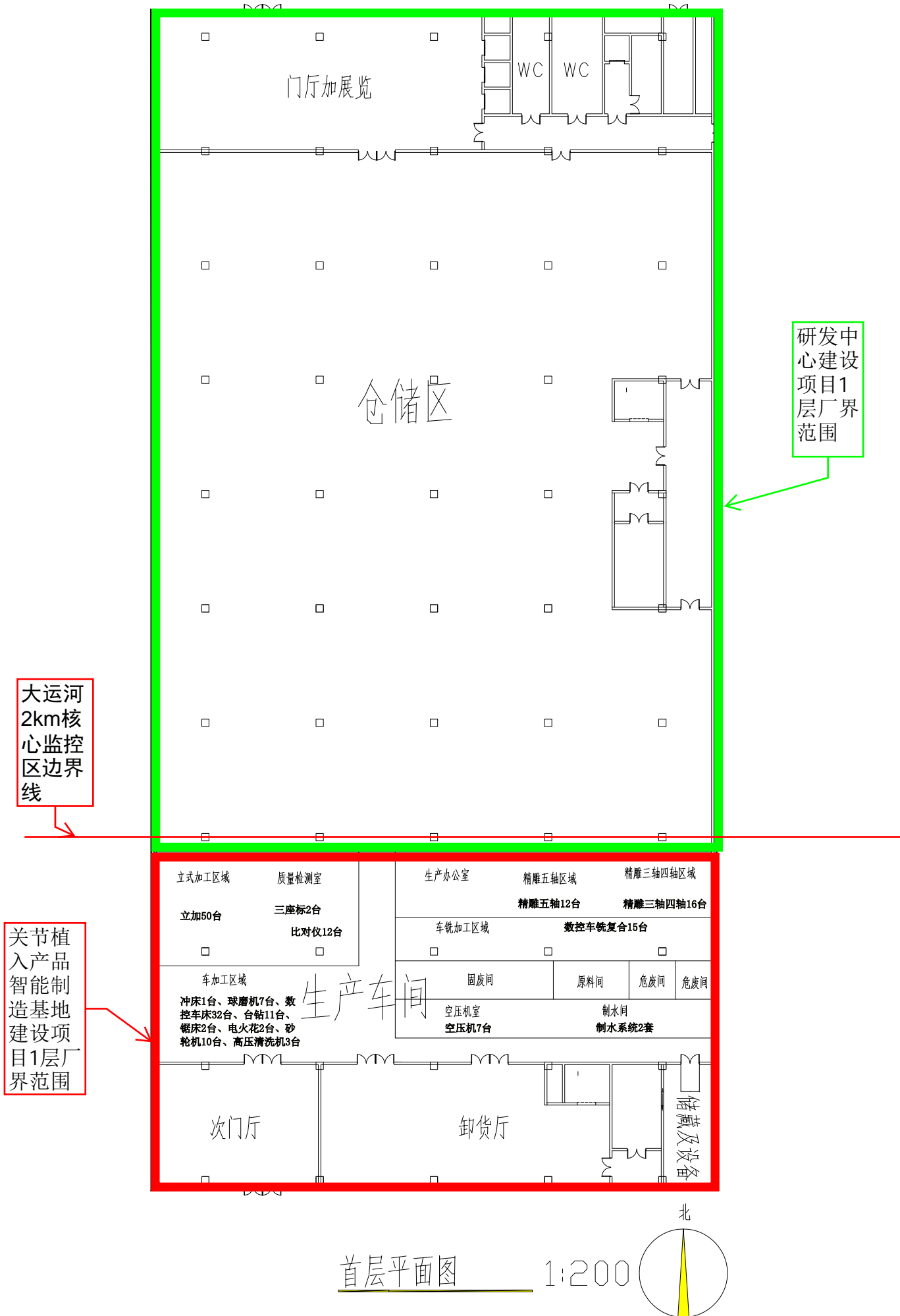
附图6-1 建设项目厂房平面布局图-1F
