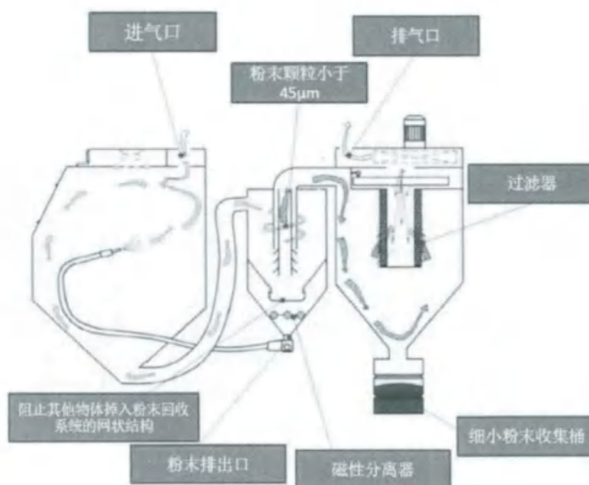
图 2-4 粉末回收系统处理工艺图
