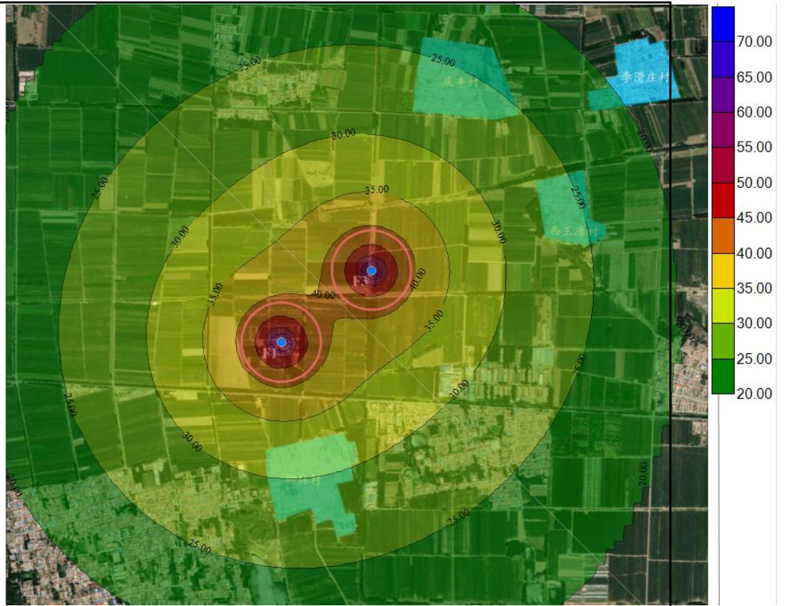
图 4-2 本项目噪声预测等声级线图 (F1、F3 风机)
