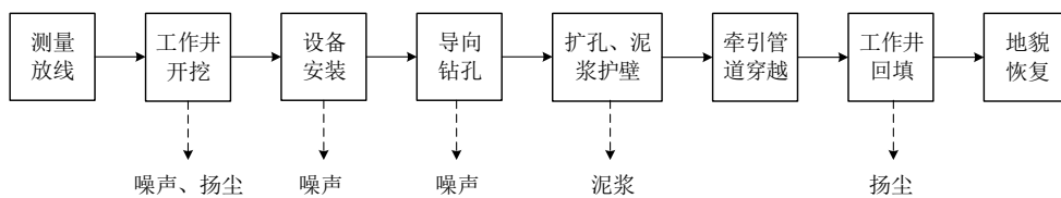
图 2-8 拉管施工产污节点图
