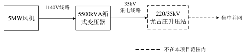
图 2-2 风力发电传输并网图
