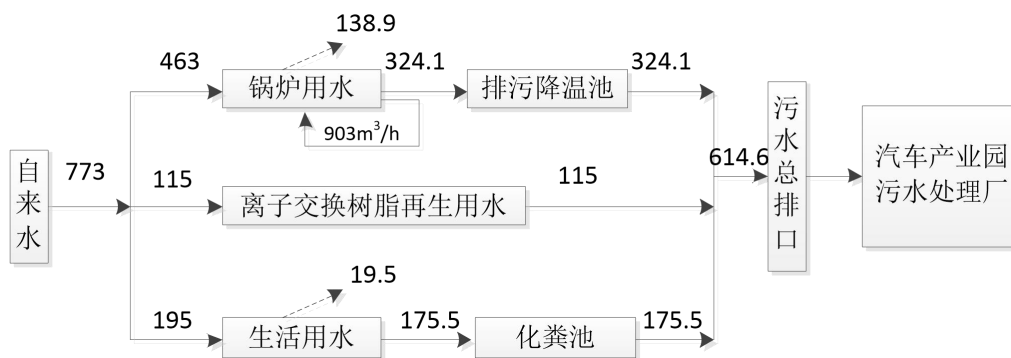
图 2-1 煤改燃后全厂水平衡图（单位：m 3 /a）
