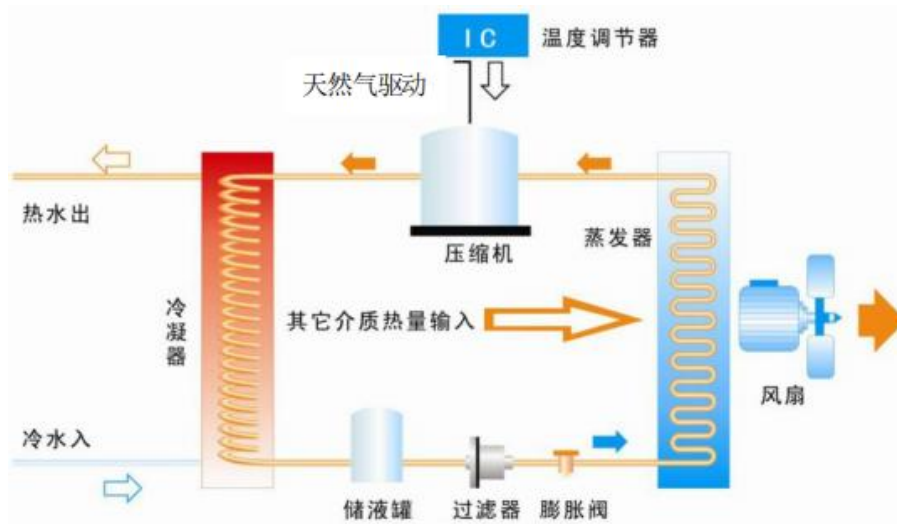
图 2-3 燃气空气源热泵工作原理图
