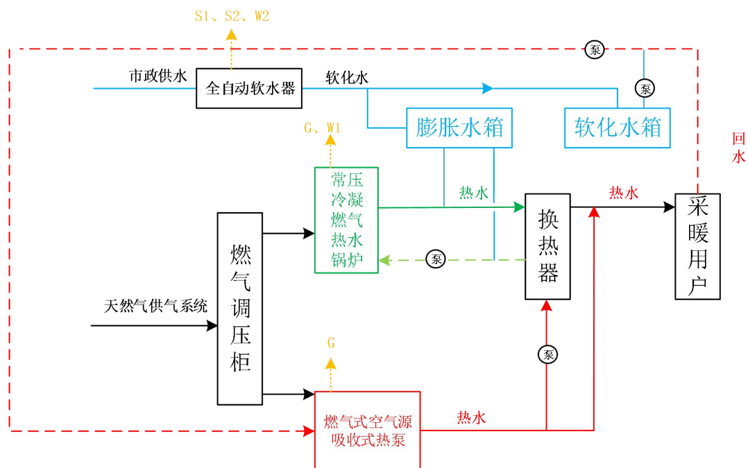
图 2-2 运营期工艺流程及产污环节图
