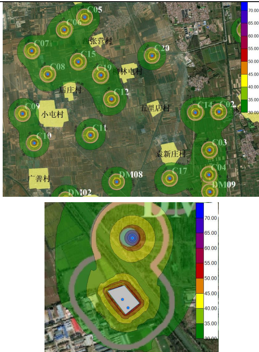
图 4-2 噪声预测等声级线图
